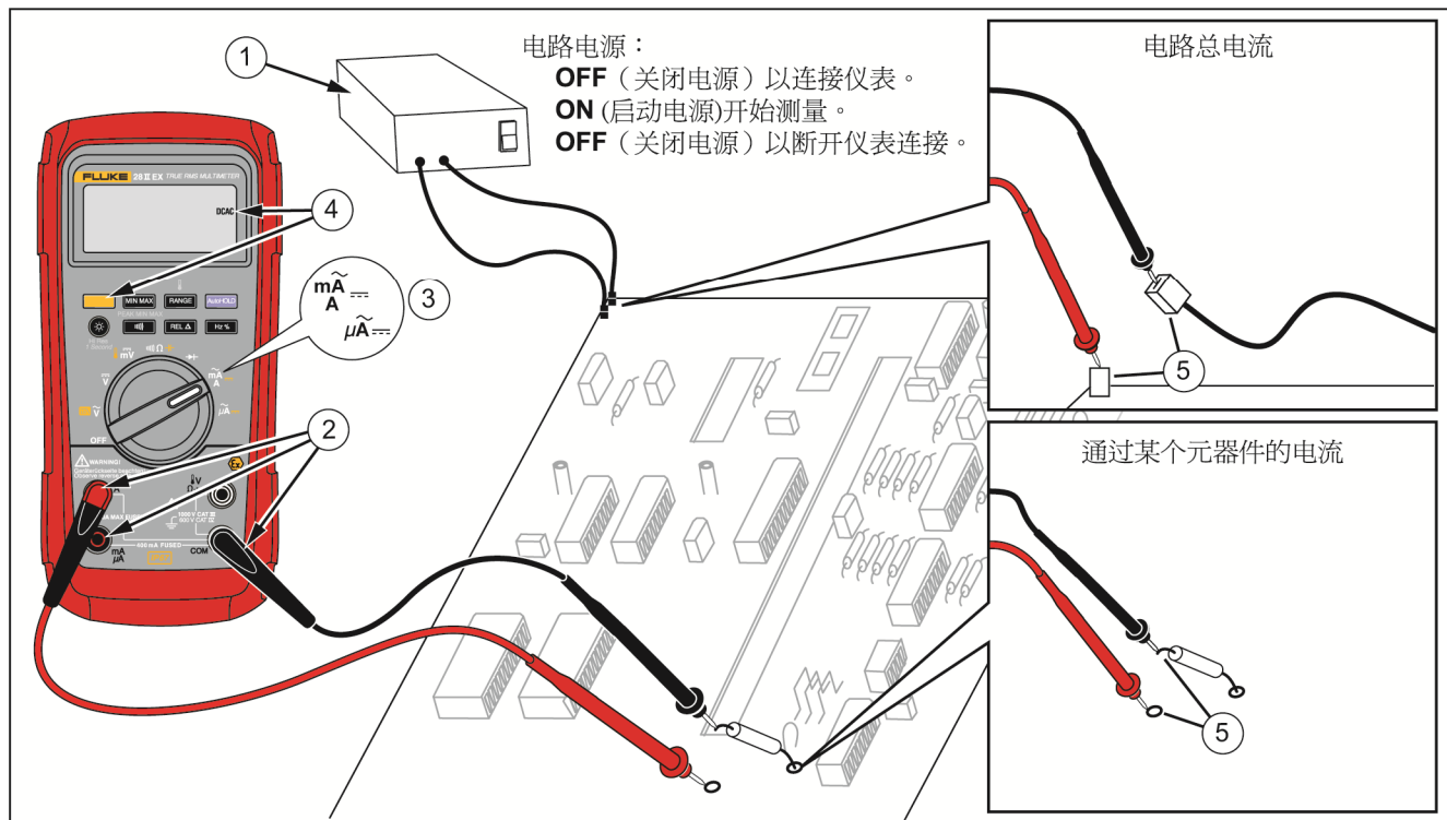
图 8. 电流测量
