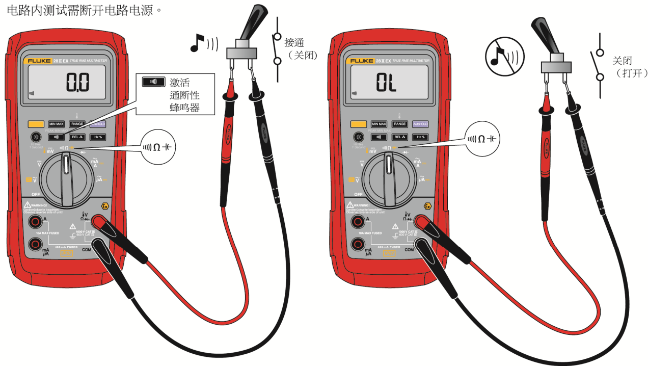
图 4.通断性测试
