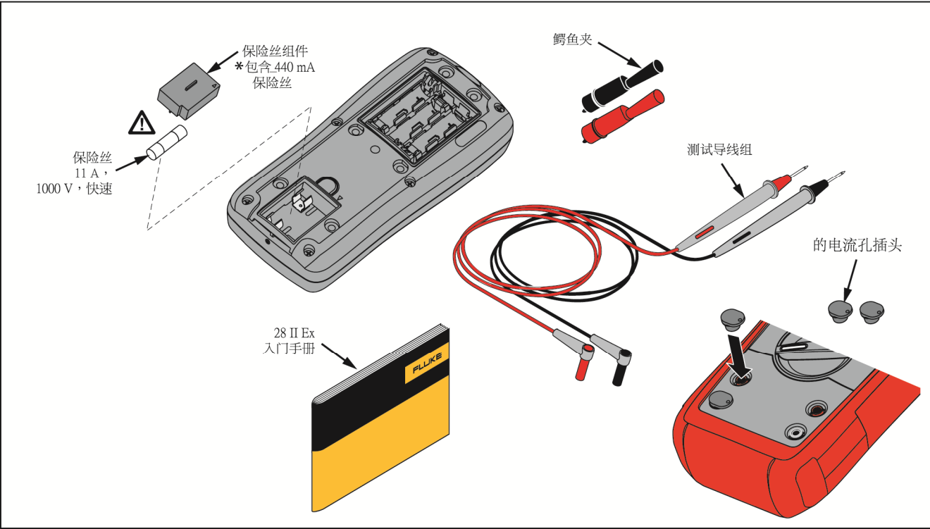
图 12.可换部件
