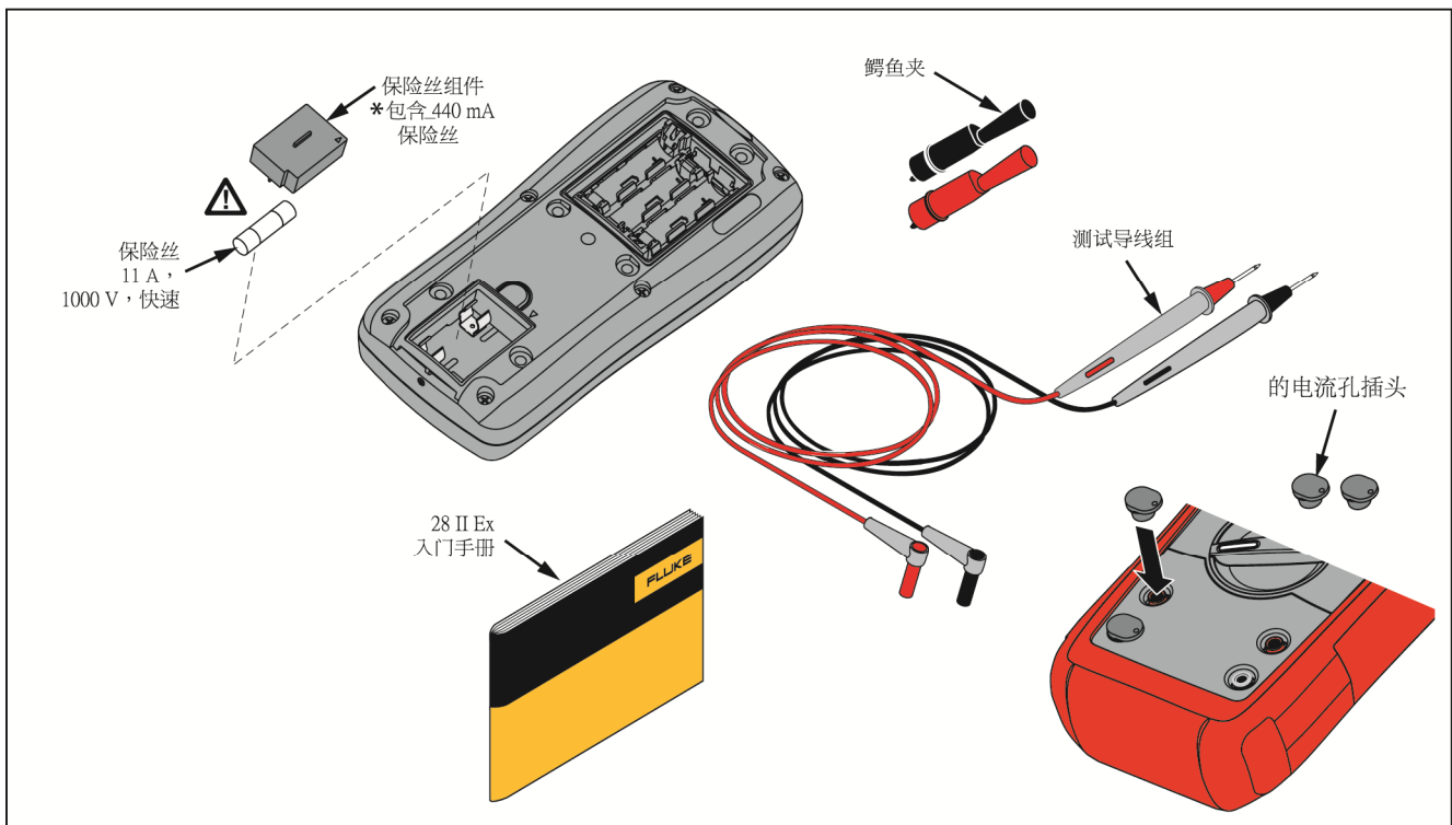
图 4.可换部件
