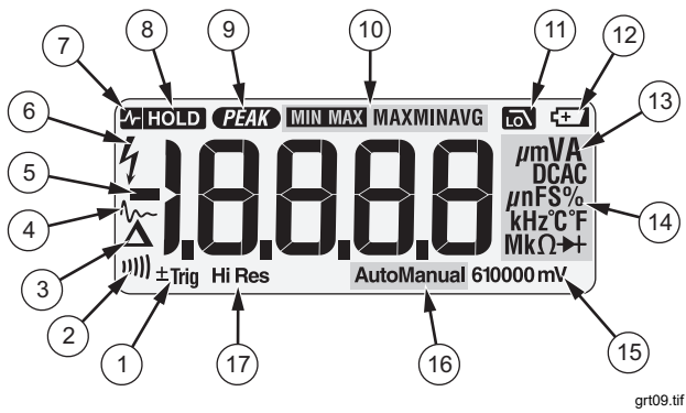
图 1.显示屏功能
