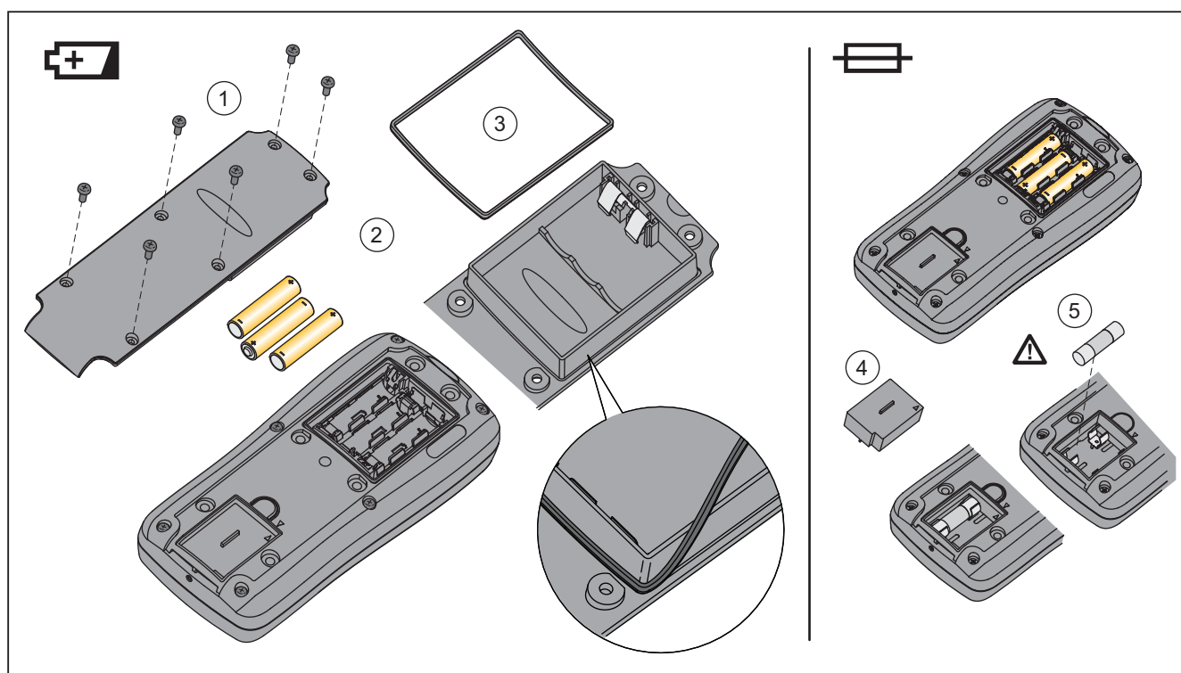
图 3. 电池和保险丝更换
