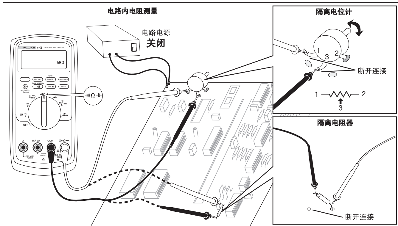
图5. 测量电阻
