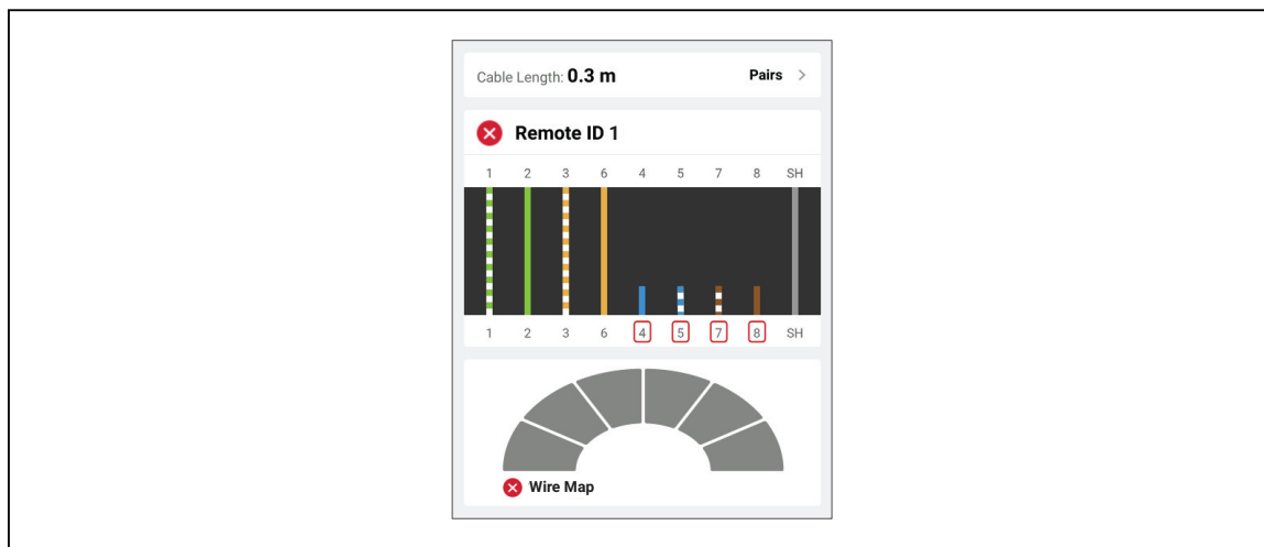
图 3. 开路线对
