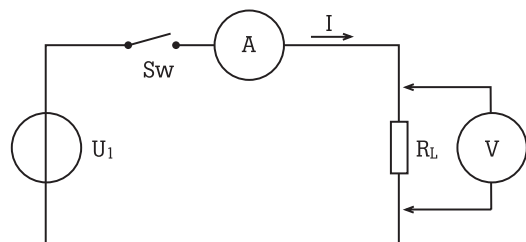
图 1. 进行电压和电流测量的基本电路。
