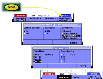
图3. 设置波形乘积的菜单结构。
