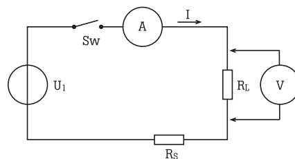
图10. 给电路增加一个电流敏感电阻来测量电流。
