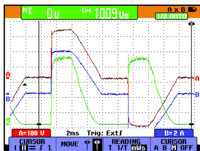
图10. 给电路增加一个电流敏感电阻来测量电流。
