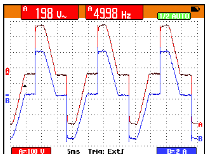
图2. 驱动一串照明灯的调光器的输出电压和电流。
