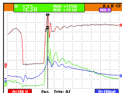
图8. 利用光标测量晶体管处理的功率的峰值。
