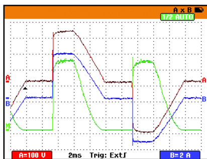
图4. Fluke 190 系列示波表上显示的电压、电流和功率曲线。
