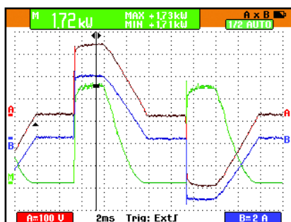
图5. 利用示波表的光标测量特定时间点的功率。
